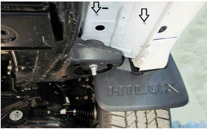
1) Vorne rechts am Fahrzeug sehen Sie die Verschraubungspunkte.
