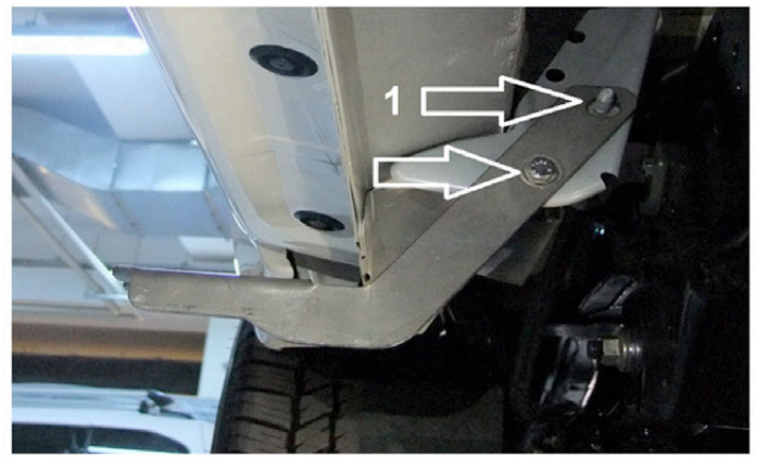
7) An der Stelle wo die 1. dargestellt wird, ist bereits eine Schraube vorhanden. Hier brauchen Sie nur die M10 Muttern und Unterlegscheiben anschrauben.
