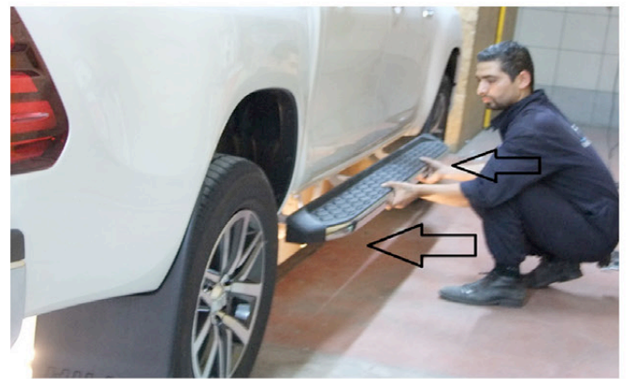
9) Als letztes montieren Sie das Trittbrett an die Halterung und befestigen Sie von unten die M8 Schrauben.
