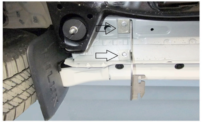
2) Befestigen Sie hier die Halterungen mit den M10 Schrauben.
